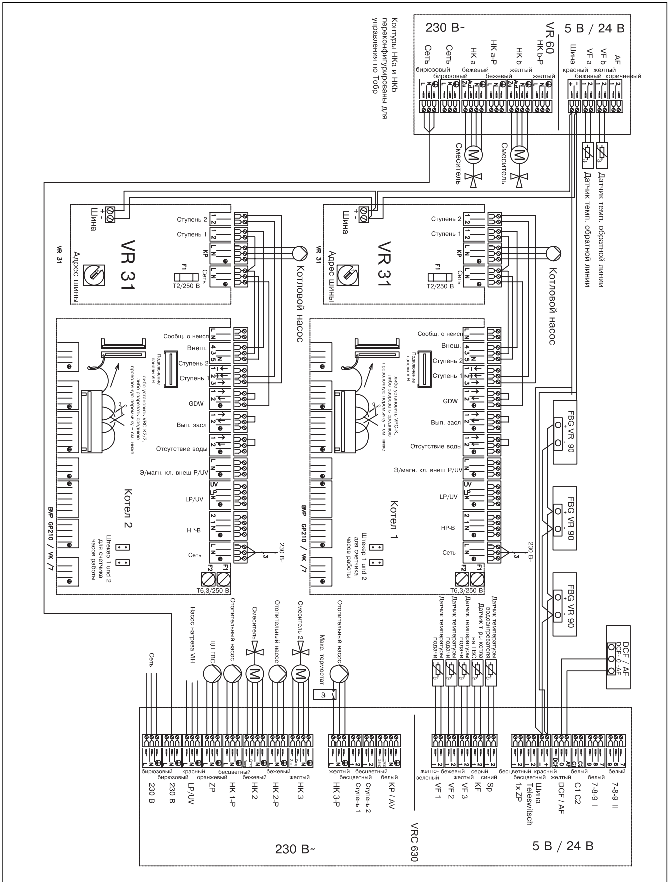
Рис. 4.15 Соединительная электропроводка VRC 630, GP210, 3 OK, VИH
