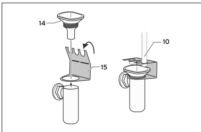
Abb. 4.2 Ablauftrichter vorbereiten
