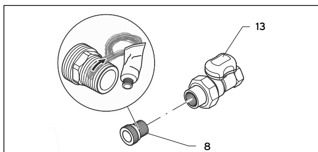
Abb. 4.4 Vorbereiten der Gasanbindung
