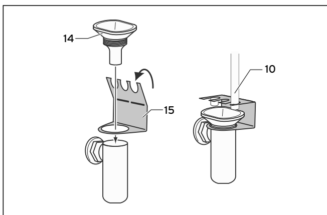
Fig. 4.2 Préparation de l'entonnoir
