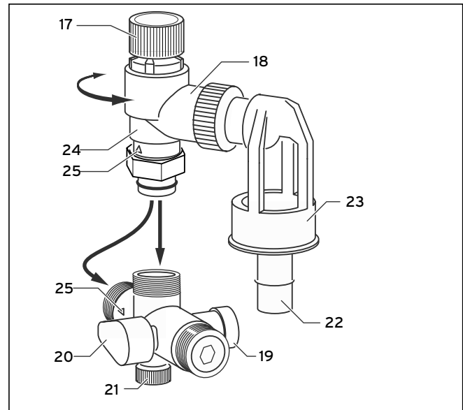
Abb. 4.5 Sicherheitsgruppe (11)
