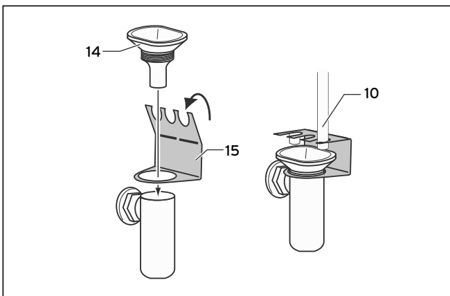
Рис. 4.2 Подготовка сливной воронки
