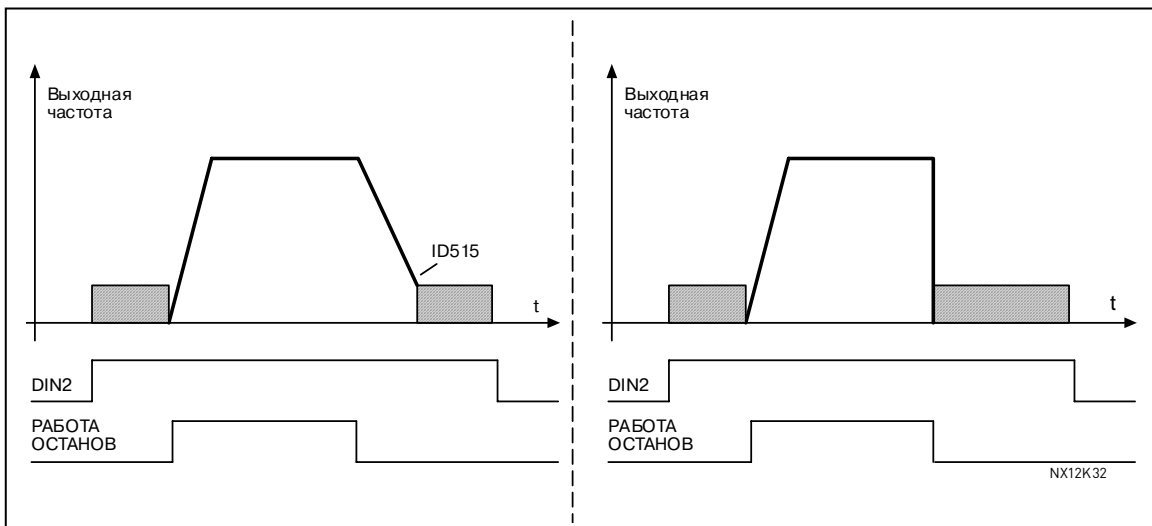
Рисунок 8-17. DIN2 в качестве входа команды торможения постоянным током (выбор 12).
