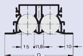
VSD35-2...4/B00
