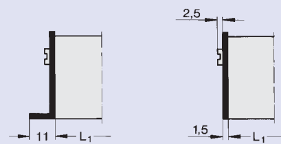
Угловая концевая заглушка
