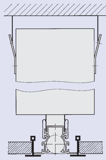
Монтаж с использованием Т-профилей
