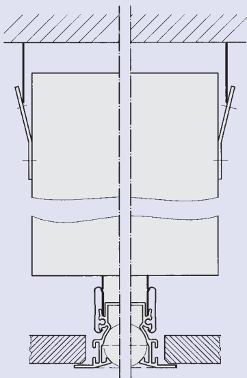
Монтаж в потолок из плит
