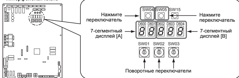
Интерфейсная плата
