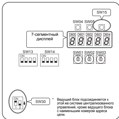
Интерфейсная плата ведущего наружного блока
