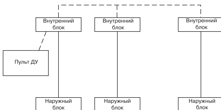
Пример группового управления блоками:
