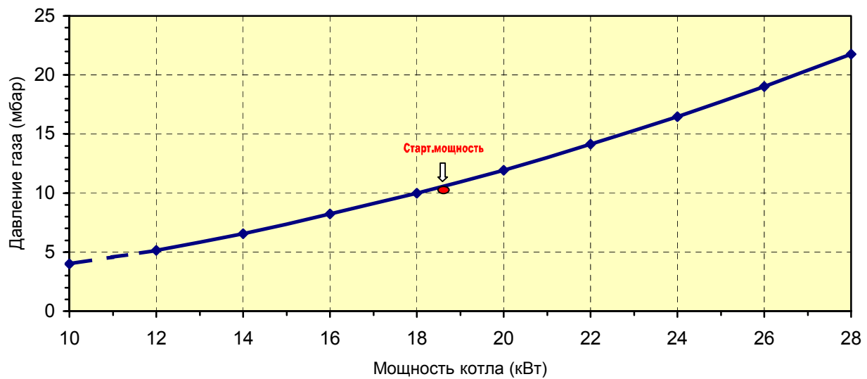
График настройки мощности THERM 28T (пропан), форсунки - 0.82 мм
