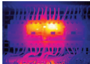
Определение перегрева электрических компонентов
