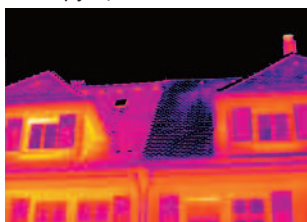
Проверка теплоизоляции в области крыш и слуховых окон
