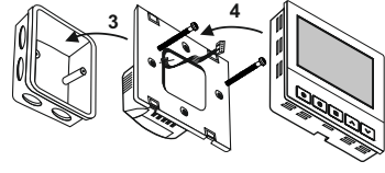
Рисунок 1 - установка термостата
