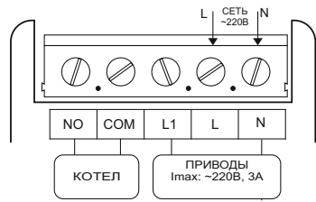
Рисунок 2 - подключение термостата
