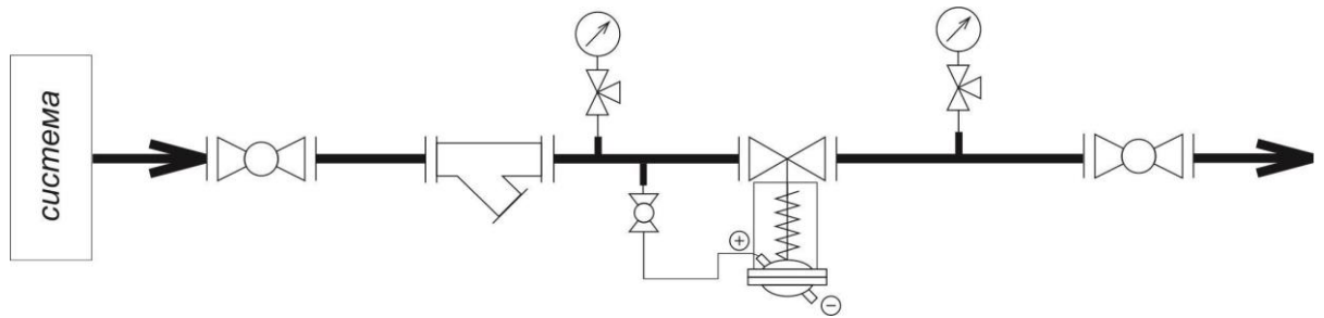
Рисунок А.2-Схема подключения регулятора
