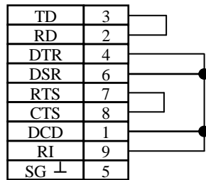
DB 9 (P) (Интерфейс RS-232)
