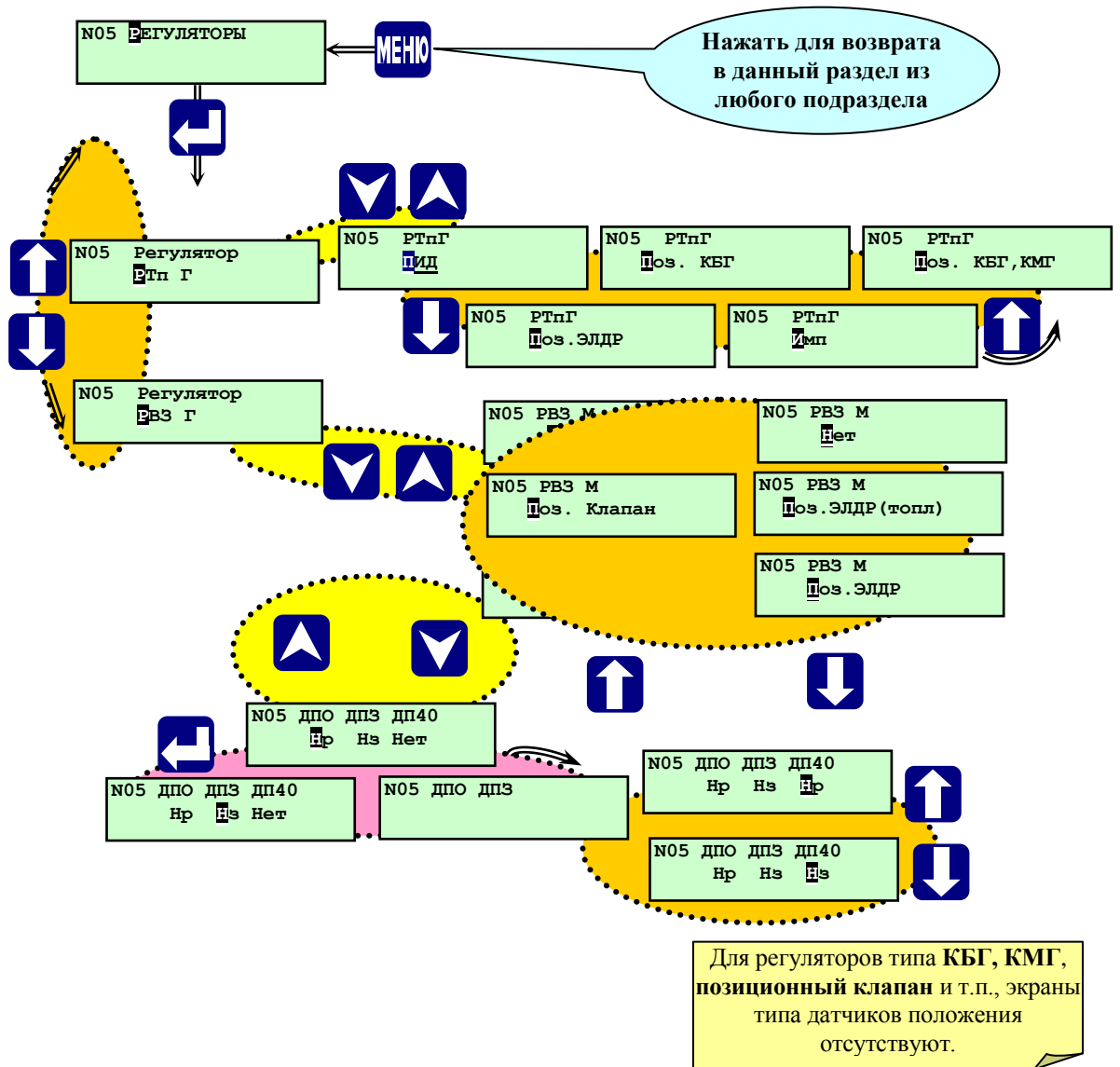
Рисунок 6.7.3.1 Раздел основного меню наладчика «Регуляторы» (водогрейный котел)
