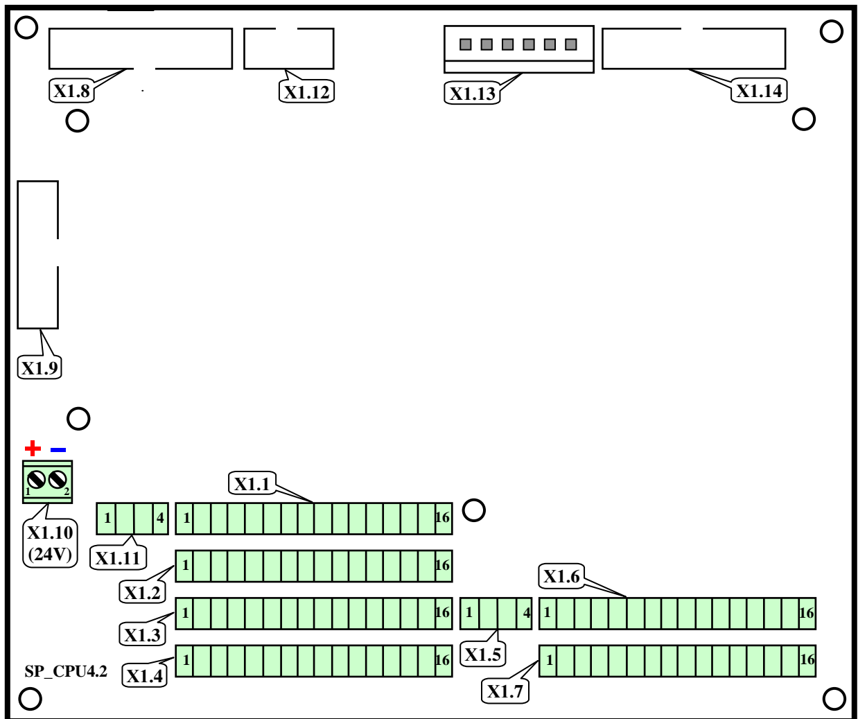
Рисунок А.2.1.1 - Расположение разъемов на системной плате SP_CPU и их нумерация, размещение платы УК (уровнемерной колонки) и нумерация её разъемов
