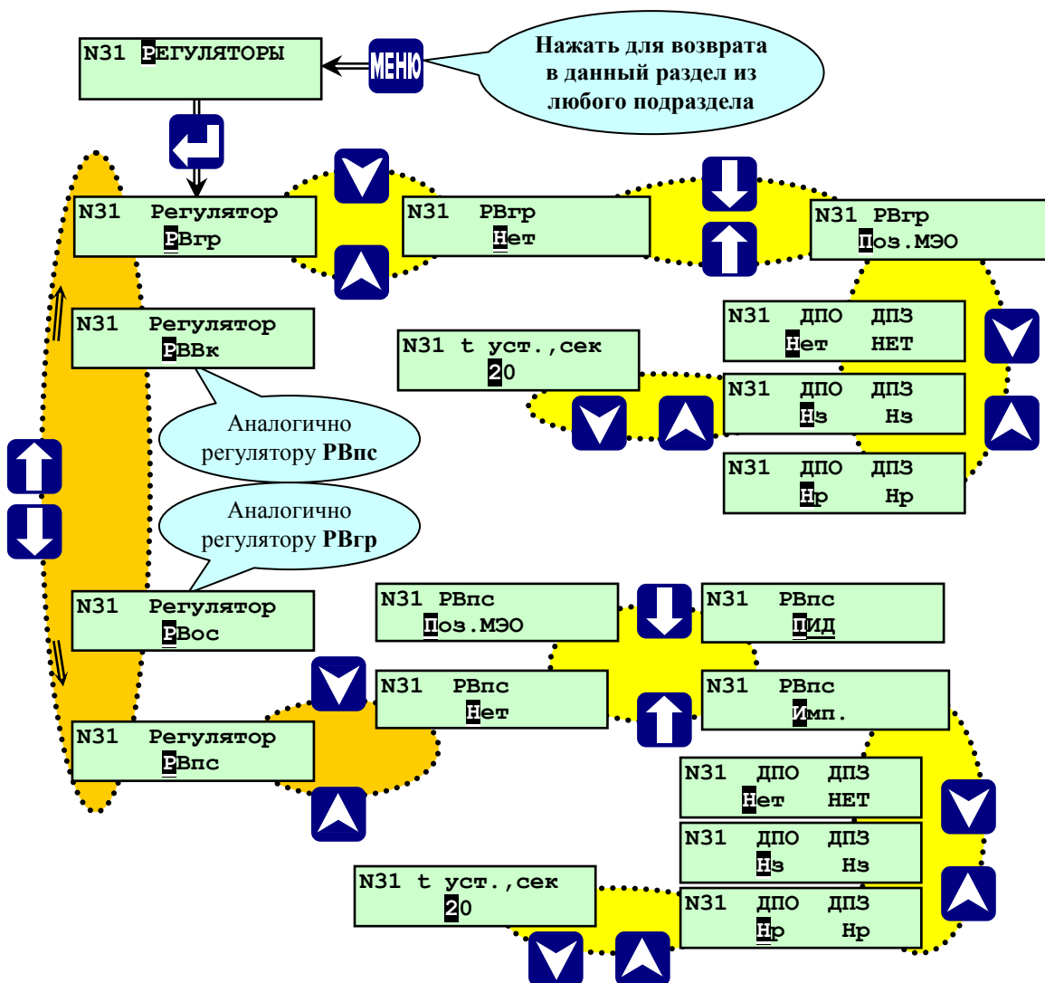
Рисунок 6.6.2.5.2- Раздел основного меню наладчика «Регуляторы»
