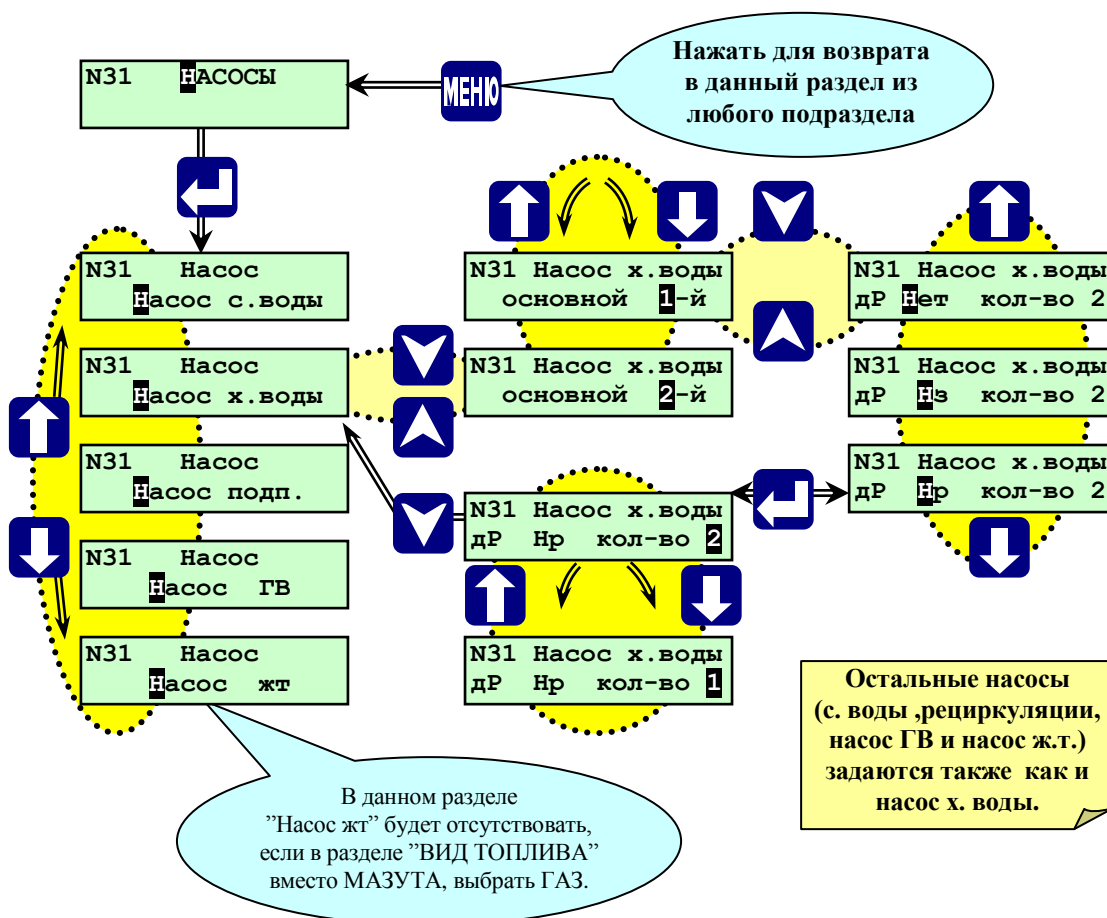
Рисунок 6.6.2.4-Раздел основного меню наладчика «НАСОСЫ»
