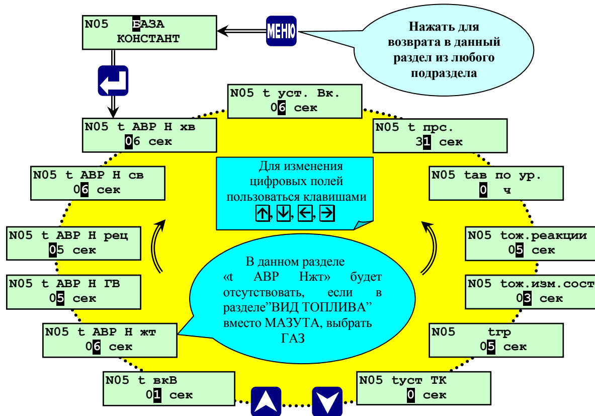
Рисунок 6.6.2.12- Раздел основного меню наладчика «База констант»
