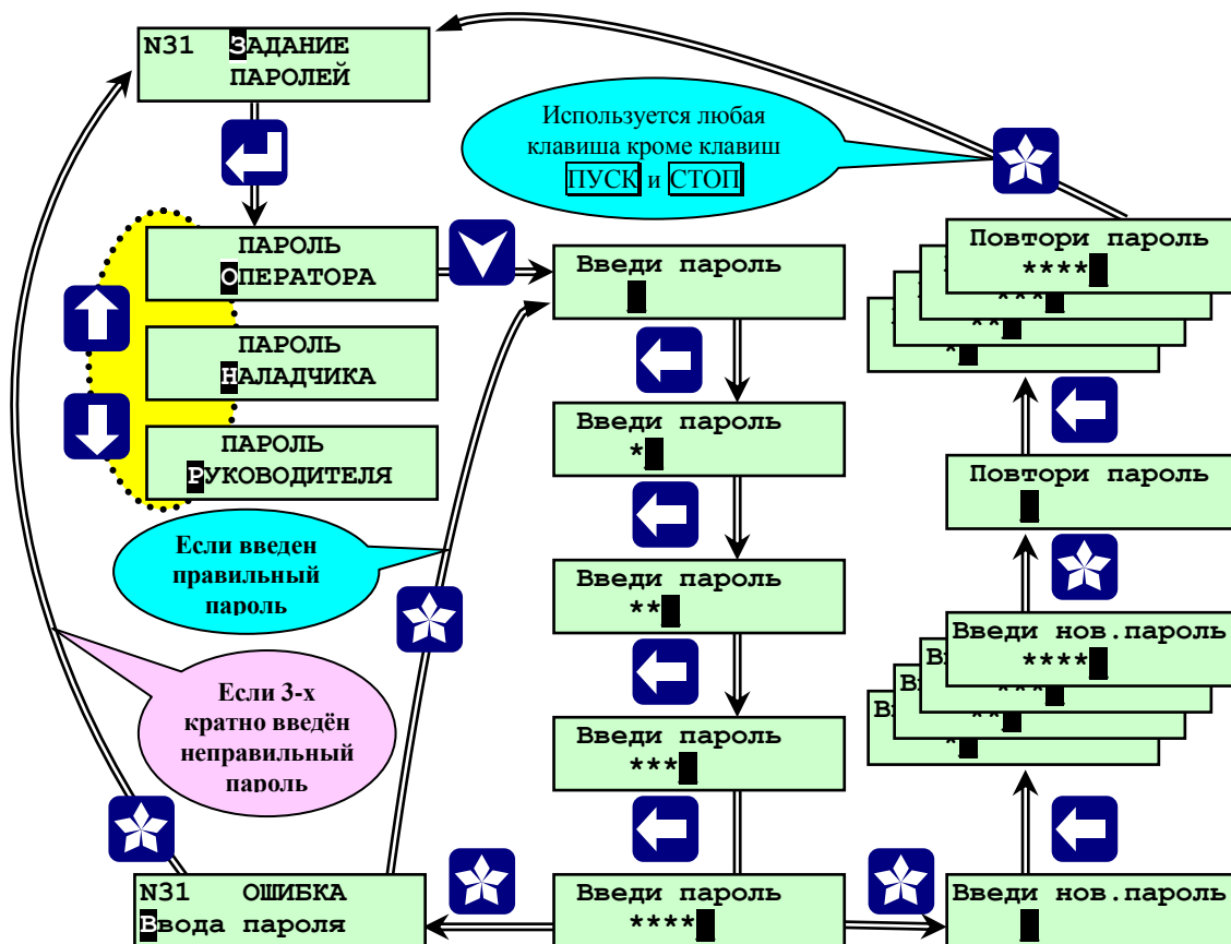
Рисунок 6.5.2.1. – Раздел дополнительного меню «ЗАДАНИЕ ПАРОЛЕЙ»
