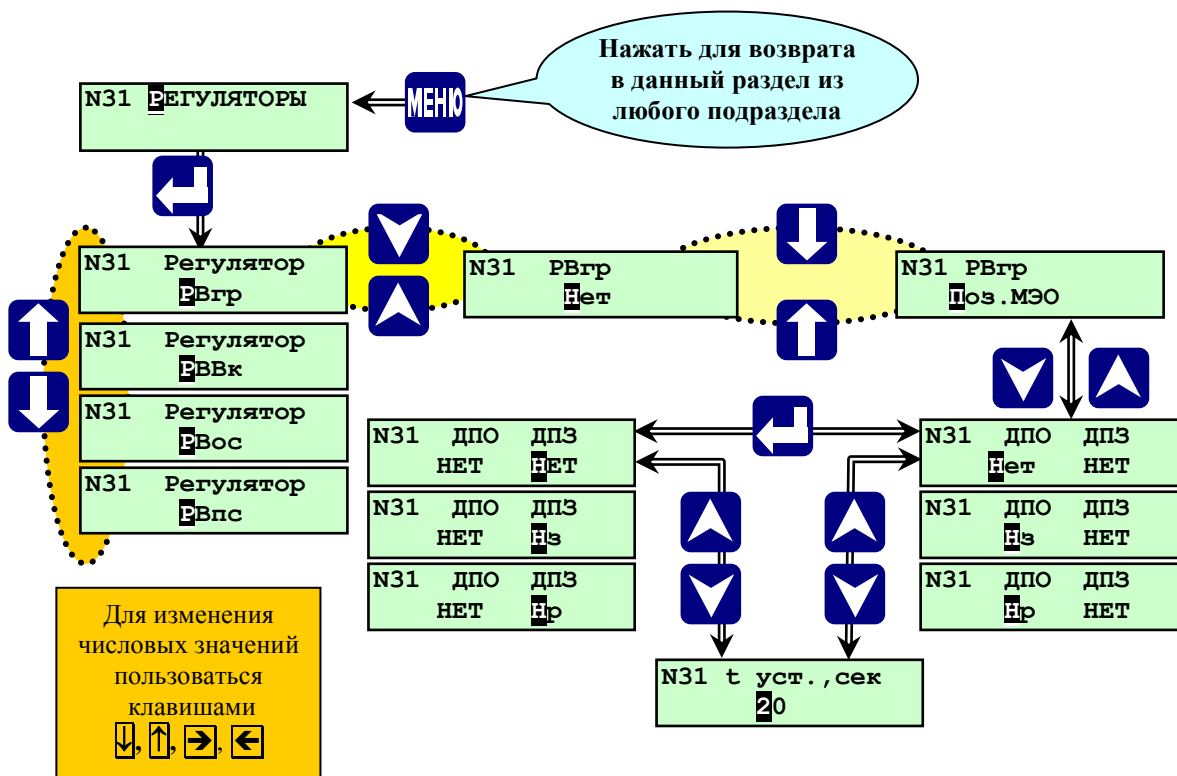
Рисунок 6.6.2.5.1- Раздел основного меню наладчика «Регуляторы»
