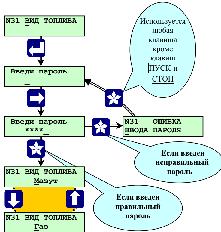
Рисунок 6.5.1.4 – Раздел основного меню оператора «Вид топлива».
