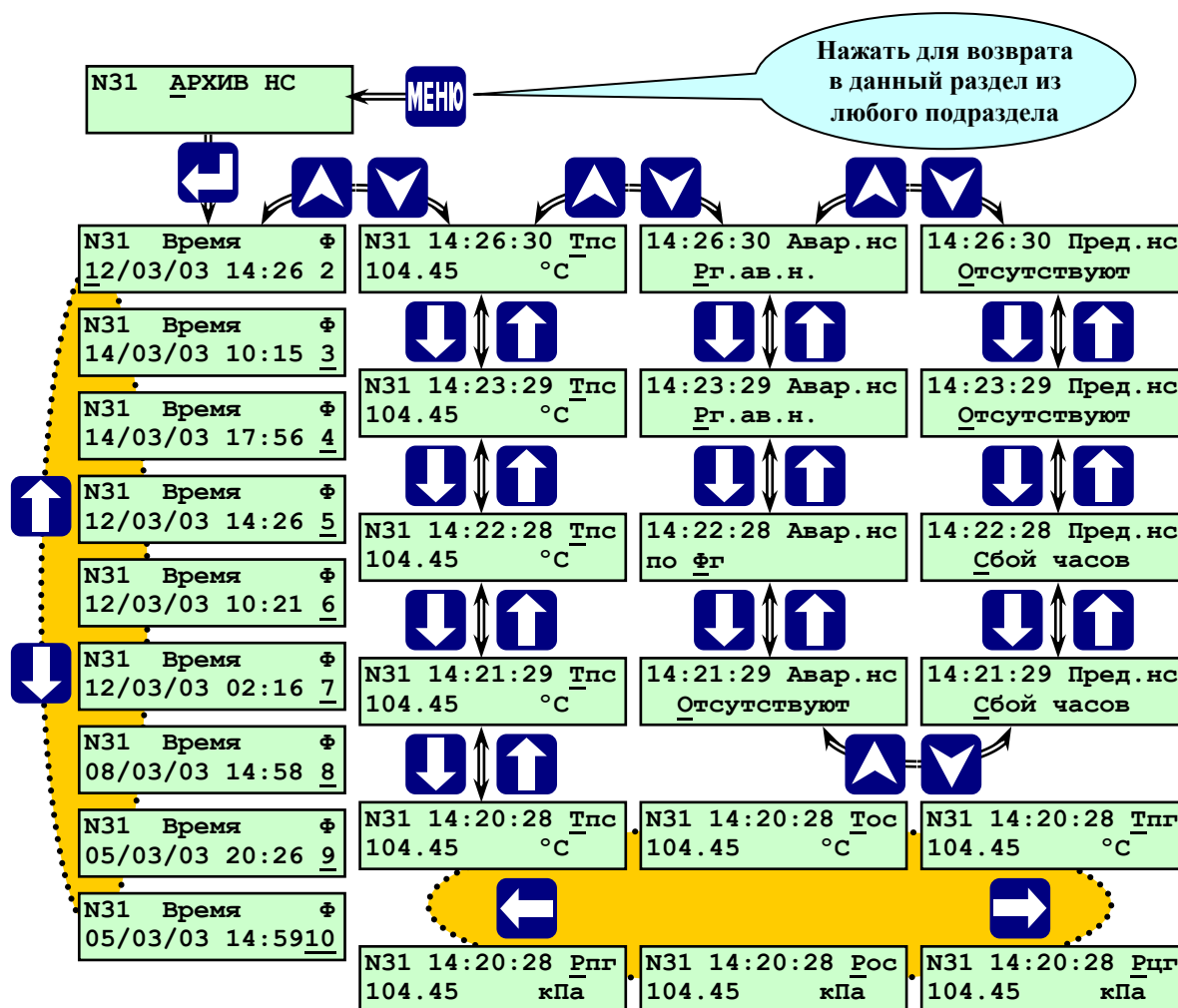
Рисунок 6.5.1.6.- Раздел основного меню оператора «Архив НС».
