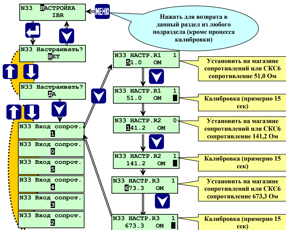
Рисунок 6.6.2.11- Раздел основного меню наладчика «Настройка IBR»
