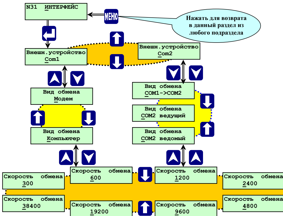
Рисунок 6.5.1.9. - Структура раздела основного меню «Интерфейс»
