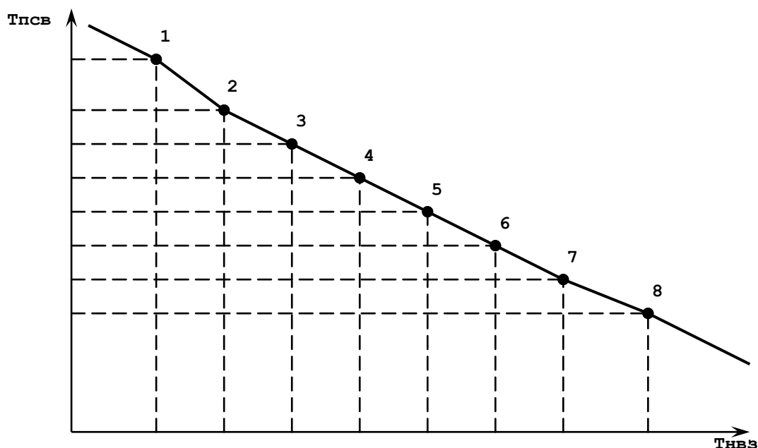
Рисунок Г.1 – Примеры задания зависимости T_{псв} от T_{нвз}
