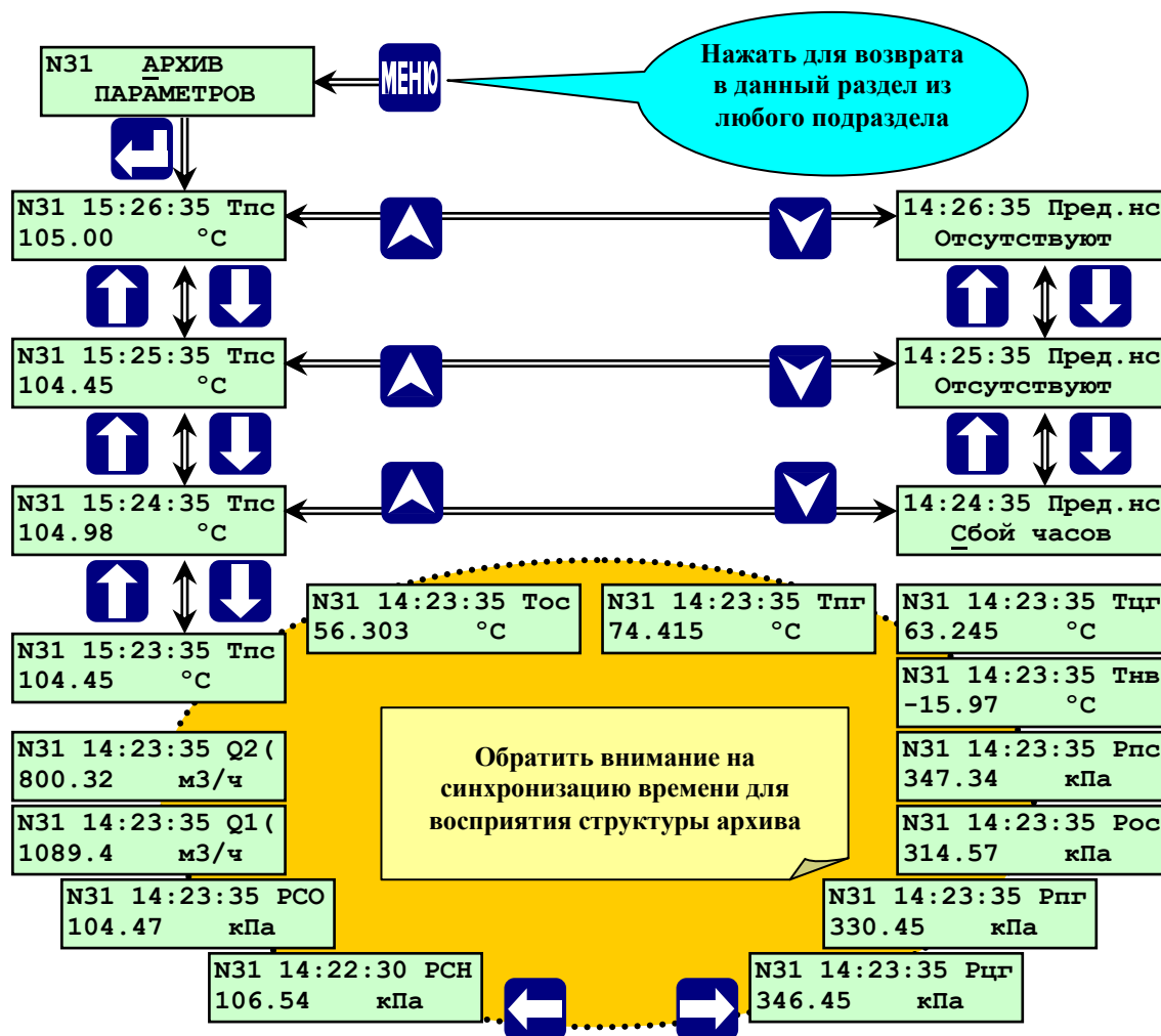
Рисунок 6.5.1.5 - Раздел основного меню «Архив параметров».
