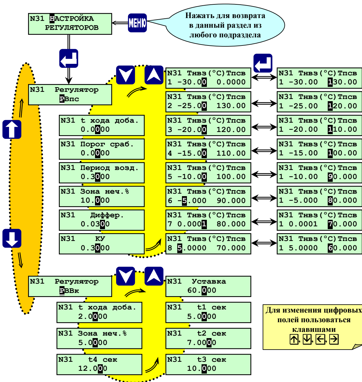
Рисунок 6.6.2.6- Раздел основного меню наладчика «Настройка регуляторы»
