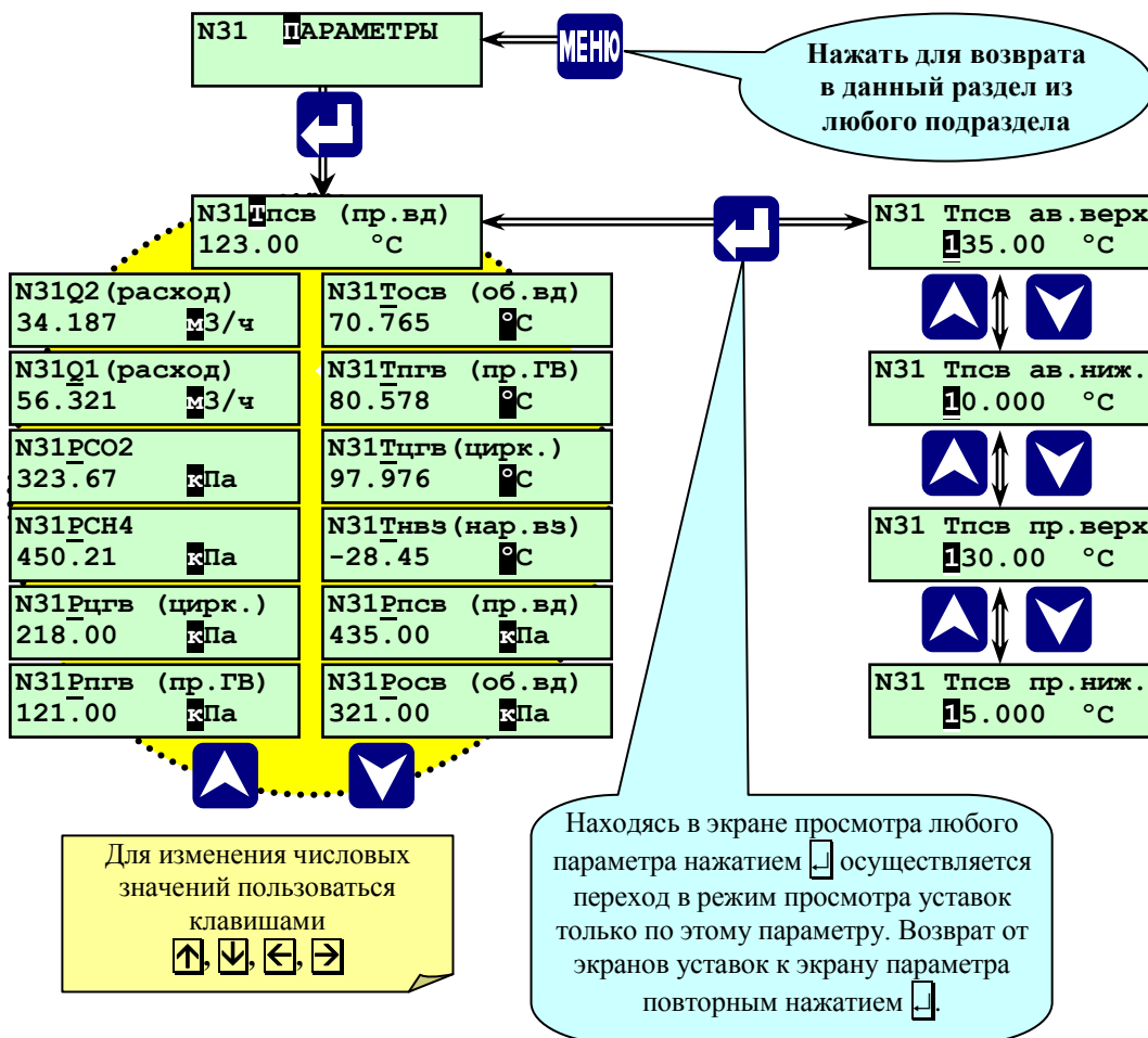
Рисунок 6.6.2.1. - Раздел основного меню наладчика «ПАРАМЕТРЫ»
