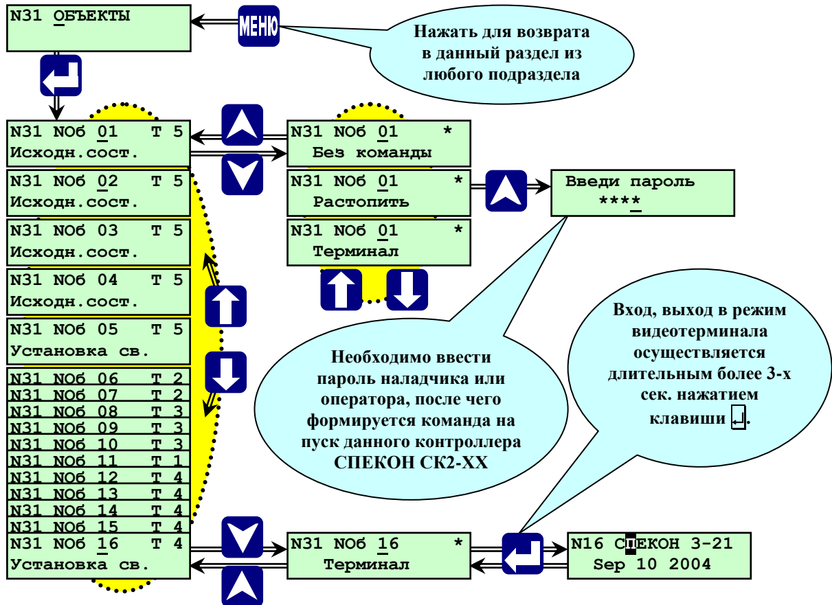
Рис.6.5.1.1.-Раздел основного меню оператора «ОБЪЕКТЫ»
