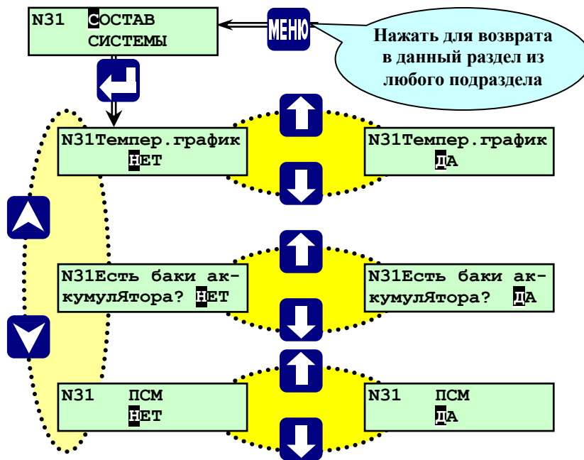
Рисунок 6.5.2.4 – Раздел дополнительного меню «Состав системы»
