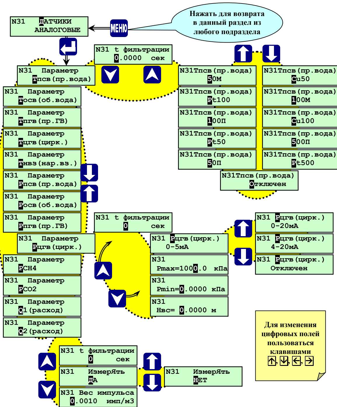
Рисунок 6.6.2.3.-Раздел основного меню наладчика «Датчики Т,Р,Н,Q»
