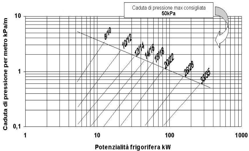
Рисунок 15: Диаграмма определения диаметра линии хладагента.
