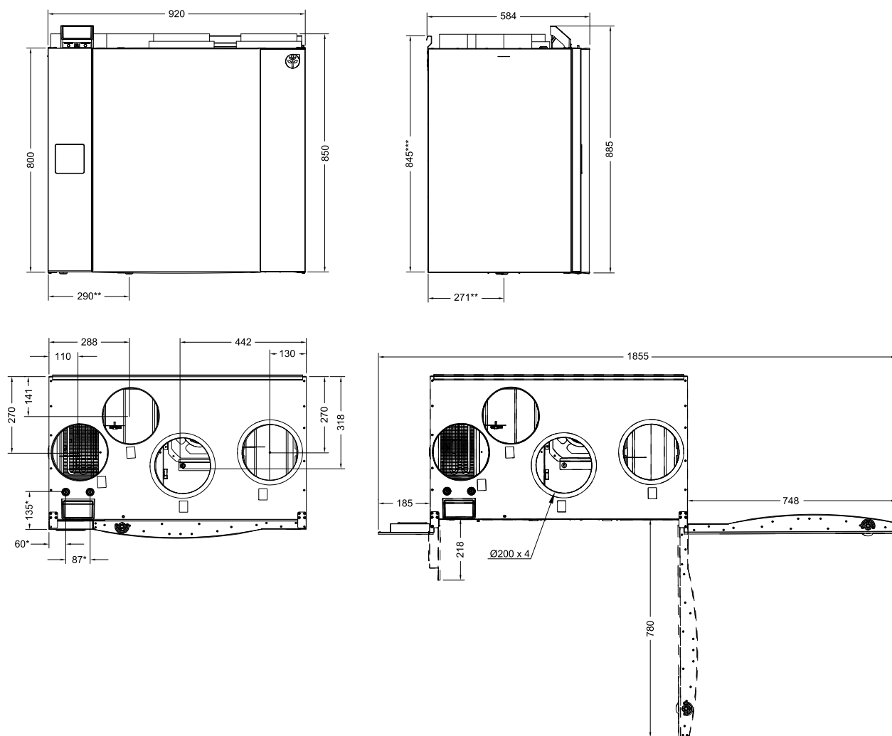
Рис. 1 Размеры и вес левосторонней модели (L)
