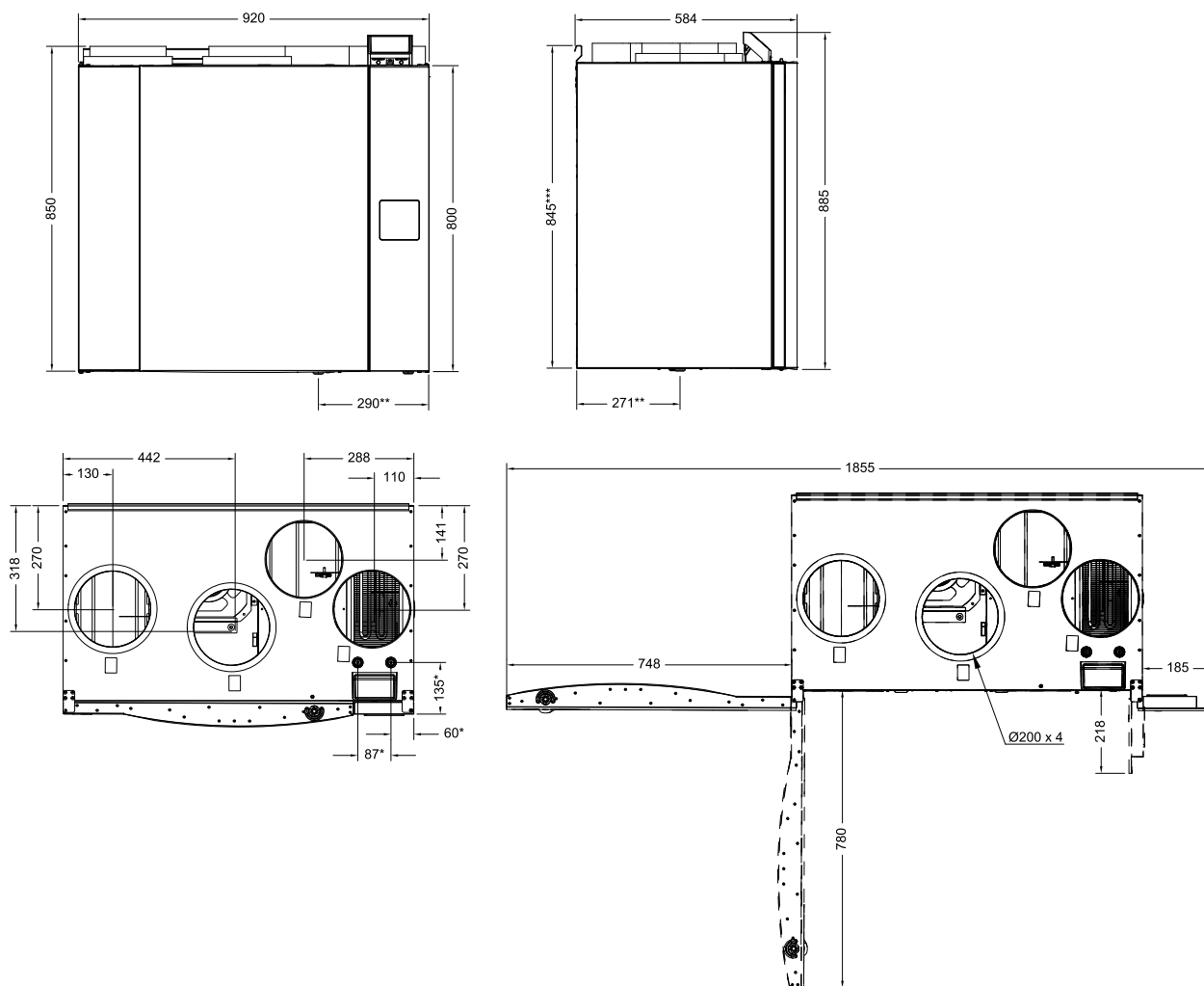
Рис. 2 Размеры и вес правосторонней модели (R)
