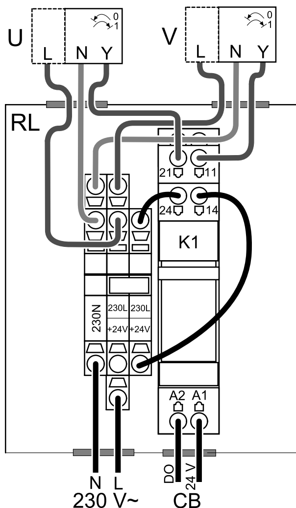
Рис. 19 Подключение клапана
