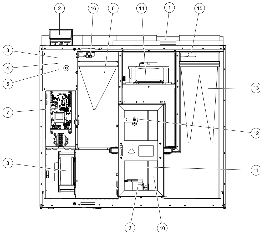
Рис. 11 Внутренние компоненты
