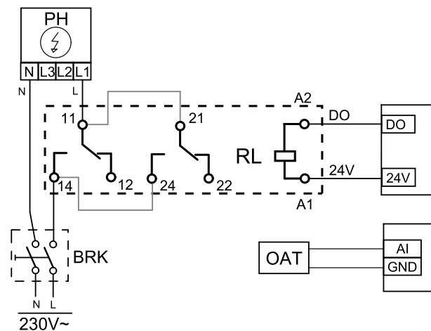
Рис. 14 Соединения предварительного нагревателя
