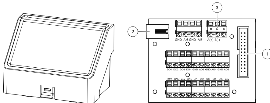
Рис. 10 Внешняя соединительная коробка и плата
