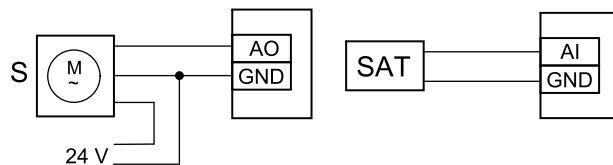
Рис. 17 Соединения каналного охладителя
