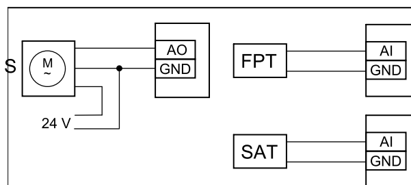
Рис. 16 Соединения водонагревателя
