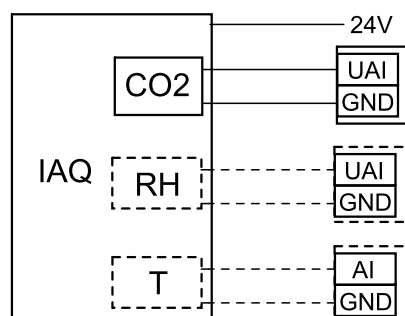
Рис. 13 IAQ соединения
