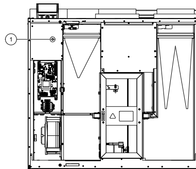
Рис. 12 Кнопка сброса защиты от перегрева
