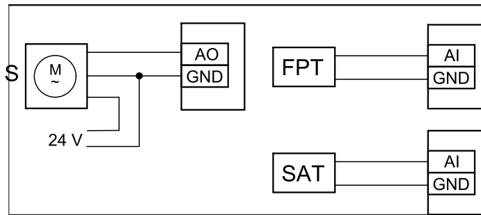
Рис. 15 Соединения водонагревателя
