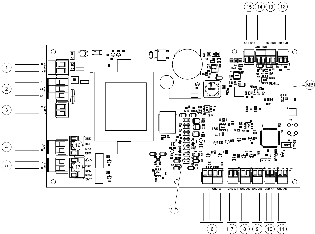
Рис. 9 Электрические соединения основной платы управления
