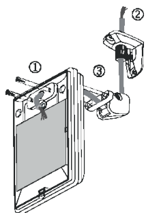
Fig.3 Installation du détecteur sur le support
