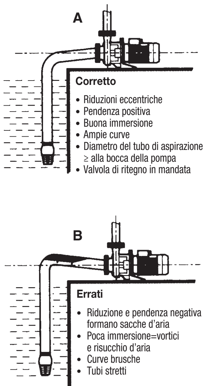
fig. 1 - schema installazione
