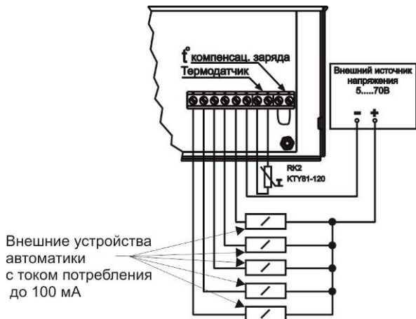
Рисунок 6 – подключение внешних устройств автоматики
