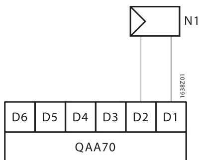
Контроллер N1 с комнатным блоком QAA70
