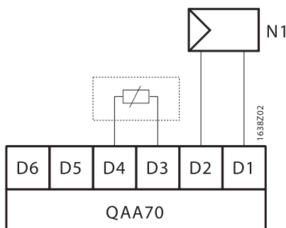
Контроллер N1 с комнатным блоком QAA70 и дистанционным датчиком (контакты D3/D4 комнатного блока)
