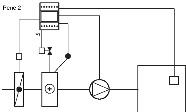
Режим Р-регулирования в помещении
