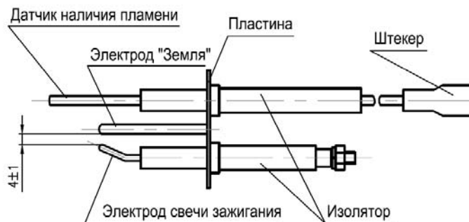
Рисунок 4.4.1 Блок розжига
