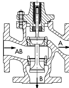
Распределительный режим трёхходового клапана Тип 3244
