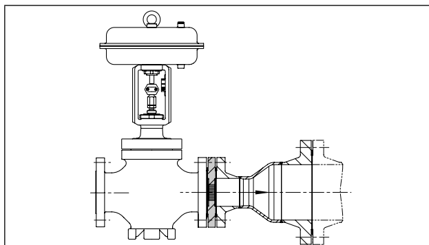
Тип 3381-1: единичная дроссельная шайба на клапане, размещаемая до возможного расширения трубопровода
