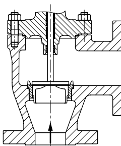
Угловой клапан Тип 3256
