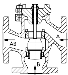
Смесительный режим трёхходового клапана Тип 3244
