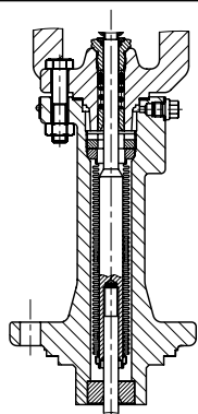
Металлическое сальниковое уплотнение
