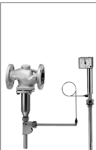
Тип 4u с регулирующим термостатом Тип 2231
