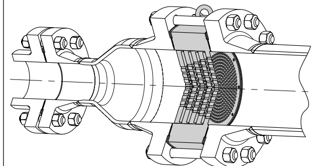
Тип 3381-4-5: пять дроссельных шайб между расширением трубопровода и трубопроводом ("слоёная" конструкция для зажима между фланцами)
