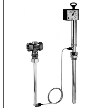
Тип 1 с регулирующим термостатом Тип 2231
