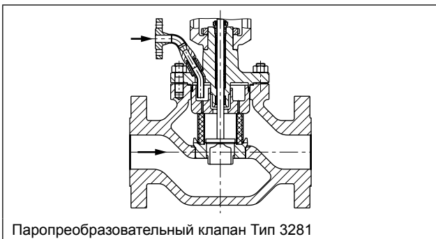
Паропреобразовательный клапан Тип 3281
