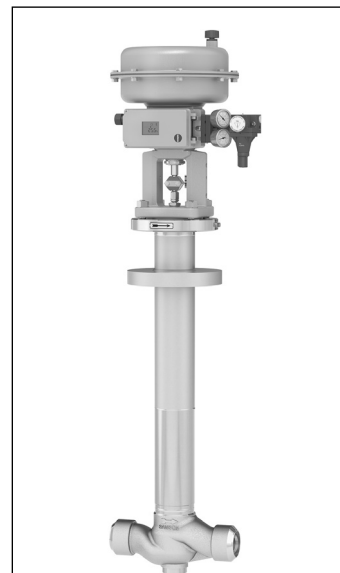
Проходной клапан из стали Тип 3248-7 с позиционером и регулятором давления
