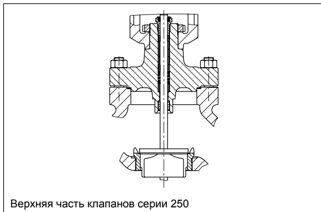
Верхняя часть клапанов серии 250
