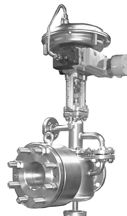
Тип 3381, прифланцованный к регулирующему клапану с обогревающей рубашкой
