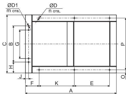
Сварная рама 4,5-11,2
