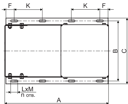
Оцинкованная рама 2,2-4,0
