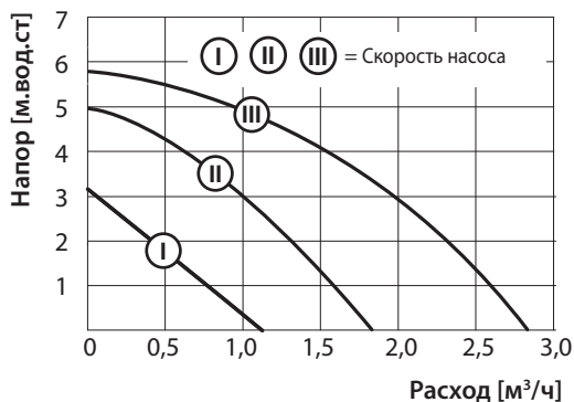
Переключение скорости насоса
