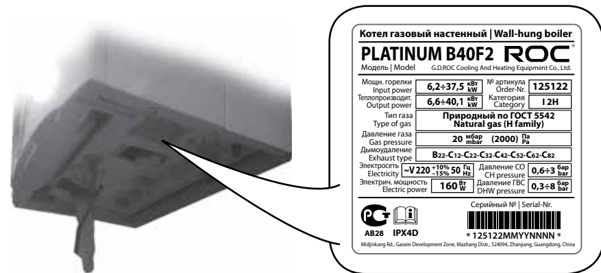
Расположение и пример шильдика котла
