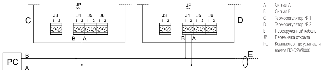
Рисунок 4.1 Схема соединения сети Modbus
