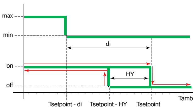
Рисунок 7.4 Схема работы в дистанционном режиме независимом/с контролем (вкл/выкл или модулирующем)
