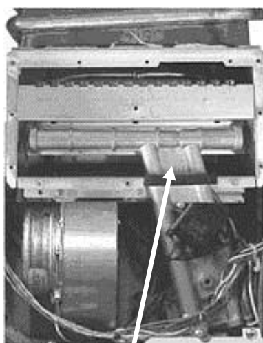
Газовый коллектор
