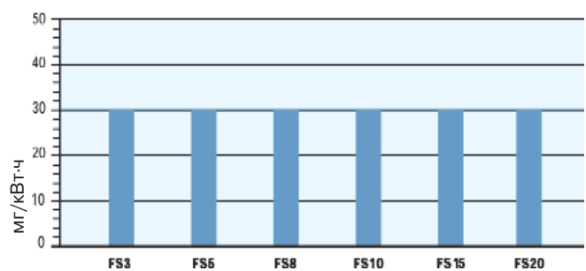
Выбросы CO
