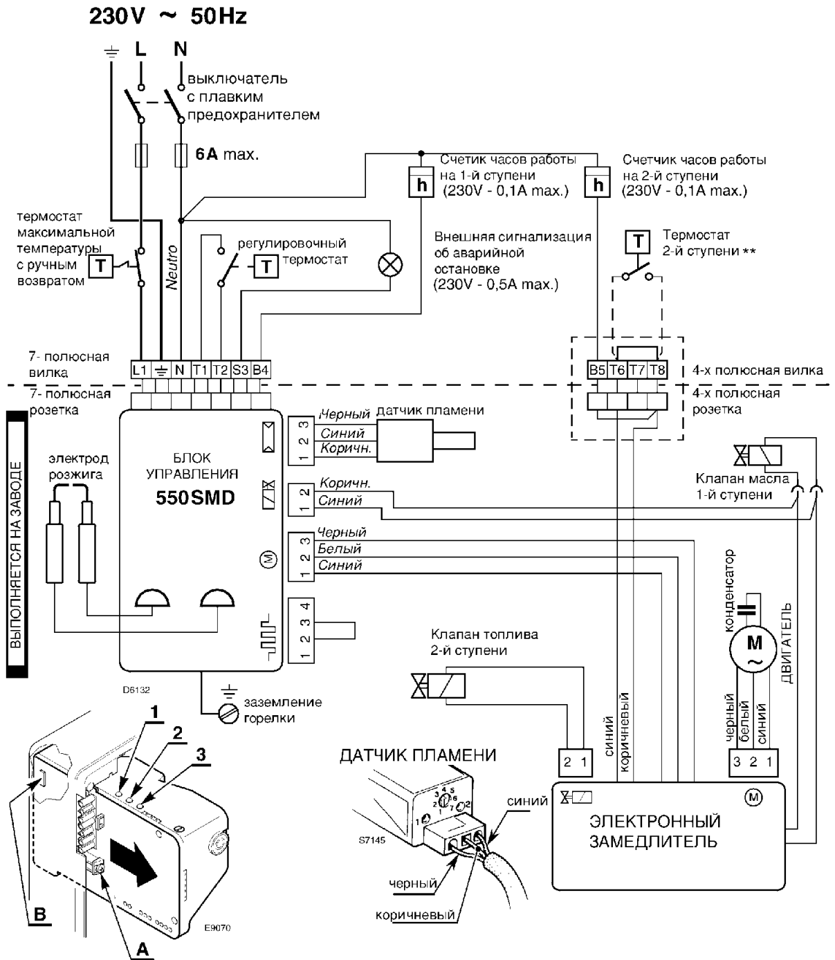
Рис. 11 (1 – Зеленый индикатор (вентилятор); 2 – Желтый индикатор (нагреватель); 3-Красный индикатор (сигнализация об аварийной остановке из-за того, что не произошло отключение)
