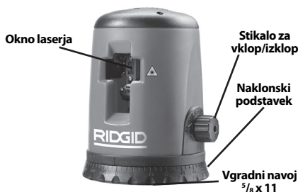
Slika 2 – Deli laserja
