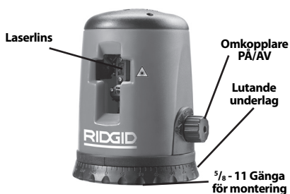
Figur 2 - Laserns delar
