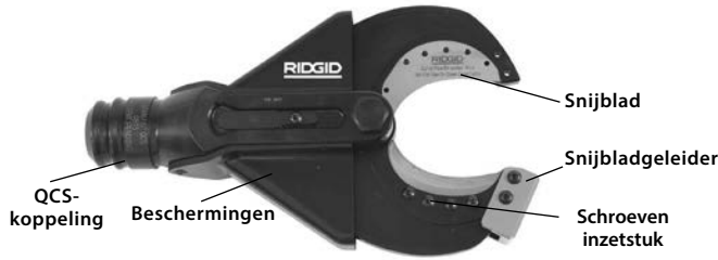
Afbeelding 1 – SC-60B Kabelsnijkop
