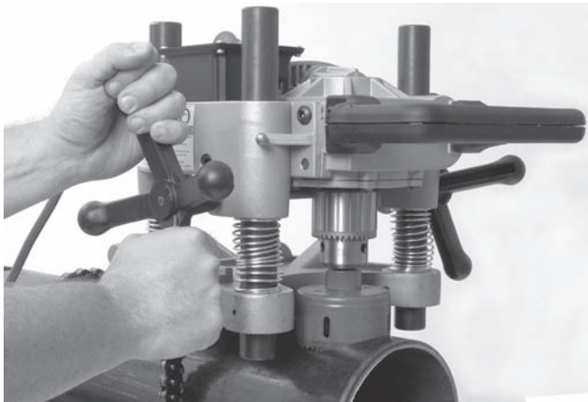
Obrázek 11 – Práce s nástrojem na vrtání otvorů
