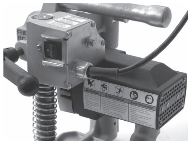
Figur 4B – Varningsetiketter på HC-300
