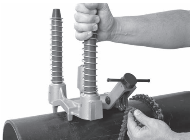
Figura 8 – Aggancio della catena
