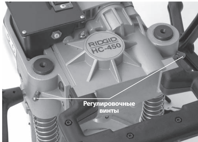
Рис. 13 – Регулировка регулировочных винтов
