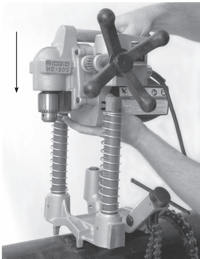
Figur 9 – Feste motorenheten til HC-300 til sokkelenheten
