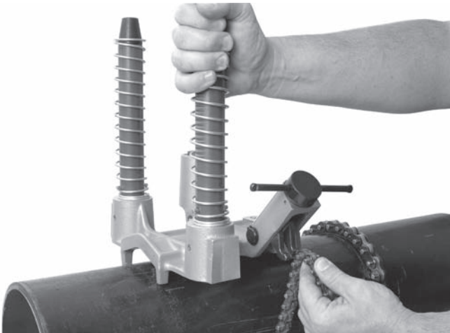
Şekil 8 – Zincirin Asılması
