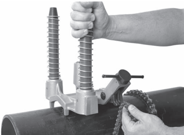
Slika 8 – Zakvačivanje lanca
