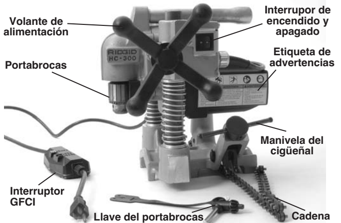
Figura 2 – Equipo estándar de la HC-300
