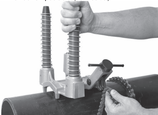
Obr. 8 – Zaháknutie reťaze
