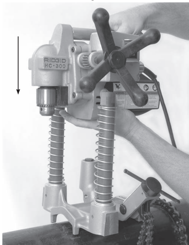
Figura 9 – Collegamento del gruppo motore dell'HC-300 alla base
