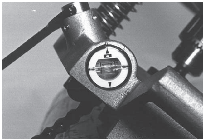
Abbildung 6 – HC-450 Wasserwaage der Lochsäge
