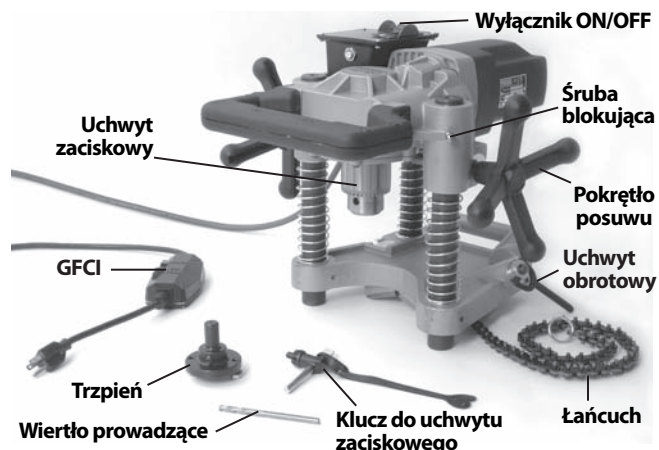
Rysunek 1 – Model HC-450 z wyposażeniem standardowym
