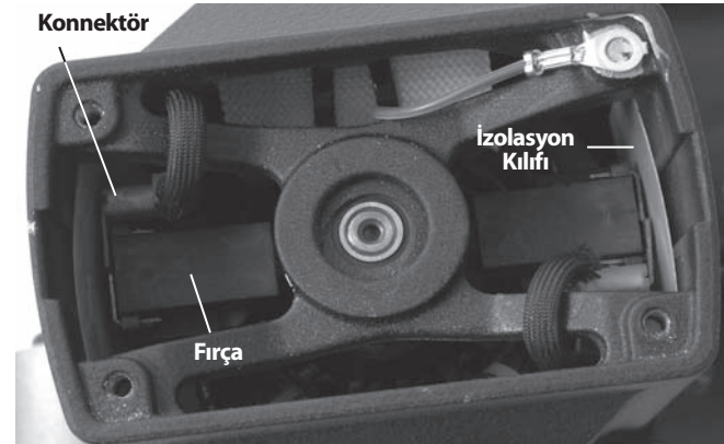
Şekil 12 – Fırça Değiştirme - Motor Kapağı Çıkarılmış Halde
