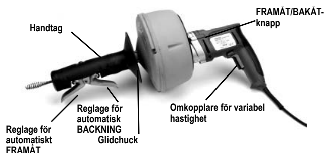
Figur 1 – K-39AF Avloppsrensare
