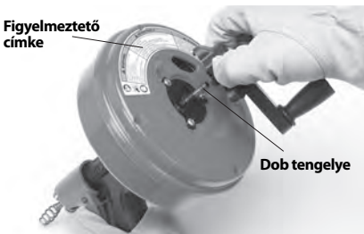
2. ábra – A forgatókart leszerelése a Power-Spin-ről
