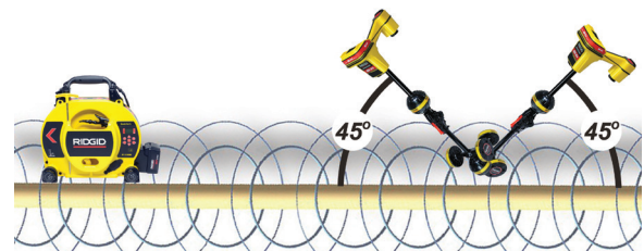
Рисунок 5 – Проверка с помощью наклона на 45°
