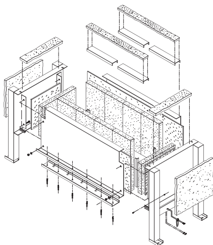
Рис. 4 Топочная камераТеплообменник
