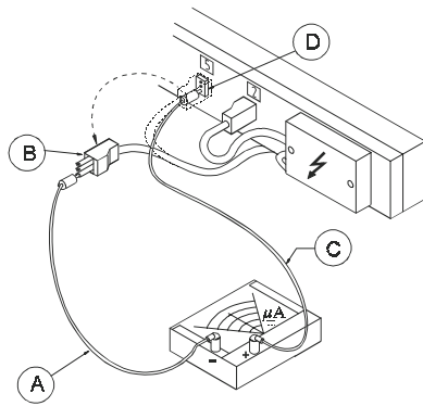
Рис. 22 Измерение ионизации
