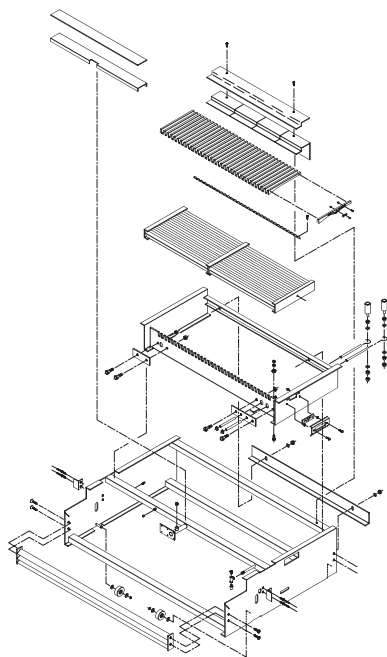
Рис. 6 Горелка
