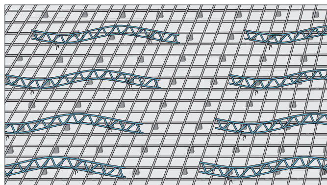
Рис. 8-26 Шаг 2: Установить S-образный арматурный каркас
