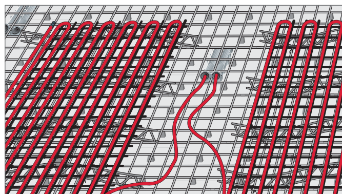
Рис. 8-27 Шаг 3: Установить модули ВКТ REHAU
