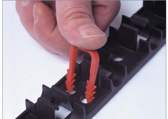
Рис. 3-35 Вдавливание гарпун-скоб в конструкцию пола
