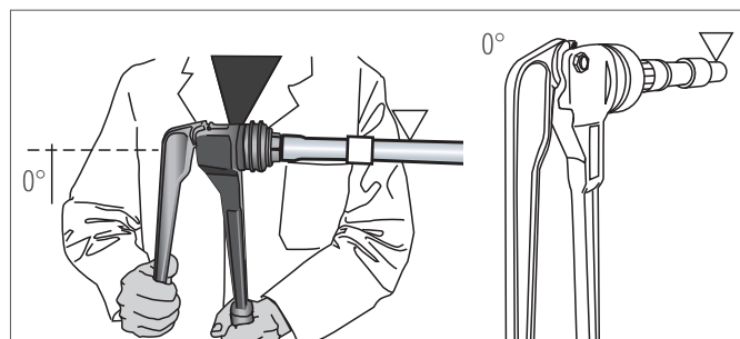
Рис. 11-5 Однократная развальцовка
