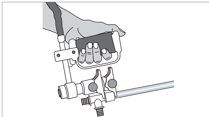
Рис. 11-9 Надвигка гильзы
