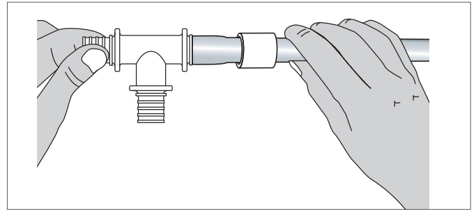
Рис. 11-7 Вставка фитинга в трубу
