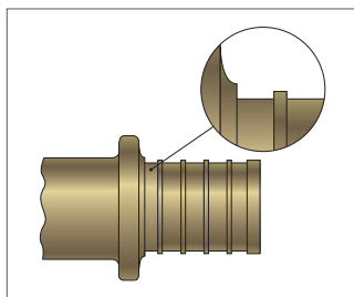
Рис. 7-7 Профиль фитингов \varnothing 40-63, RAUTITAN MX
