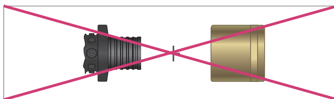
Рис. 4-7 Недопустимая комбинация фитинга RAUTITAN PX с подвижной гильзой RAUTITAN MX
