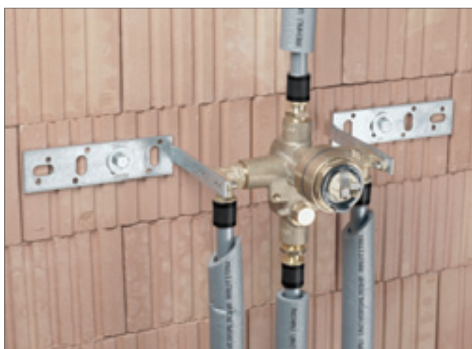
Рис. 4-11 Пример присоединения к арматуре трубами RAUTITAN
