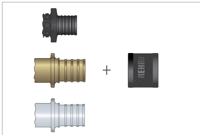
Рис. 4-6 Допустимая комбинация с подвижной гильзой RAUTITAN PX
