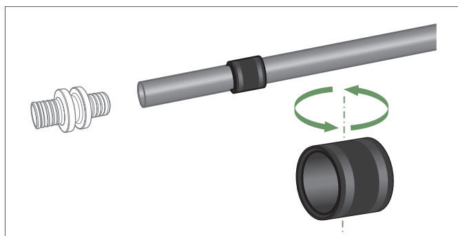
Рис. 4-8 Надвижную гильзу RAUTITAN PX можно надвигать любой стороной
