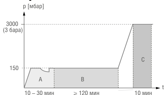
Табл. 19 Диаграмма пневматического испытания А Предварительное испытание (см. табл. 7-1) В Основное испытание С Испытание нагрузкой
