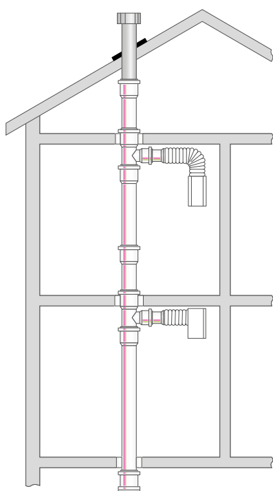
Рис. 56 Система вытяжной вентиляции из труб RAUPIANO PLUS 1 Крышный элемент 2 Гибкая подводка 3 Вытяжной вентилятор 4 Трубопроводы RAUPIANO PLUS 5 Двухраструбная муфта 6 Заглушки
