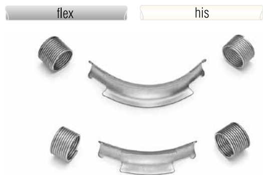
Рис. 41 Фиксаторы поворота (водоснабжение) (3–4 x Ø) – 90° или 45° для изгиба труб Ø 16–32
