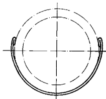
Рис. 33 Фиксирующий желоб в разрезе
