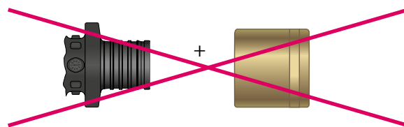
Рис. 16 Недопустимая комбинация фитинга RAUTITAN PX с надвижной гильзой RAUTITAN MX
