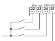
Схема разъёма цифровых вводов 230 V / AC
