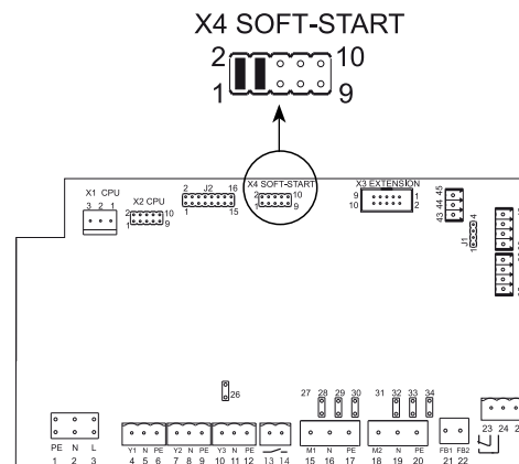
Плата вводов/выводов
