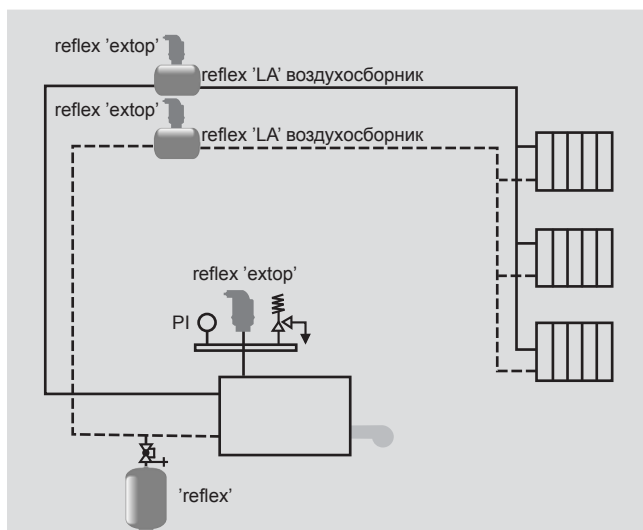
reflex 'extop' и воздушноеборник в системе после её заполнения
