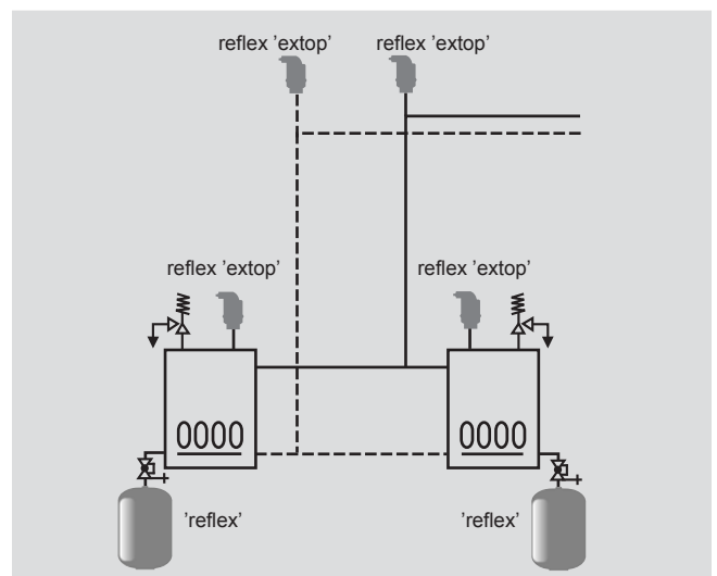
reflex 'extop' воздушной линии после её заполнения
