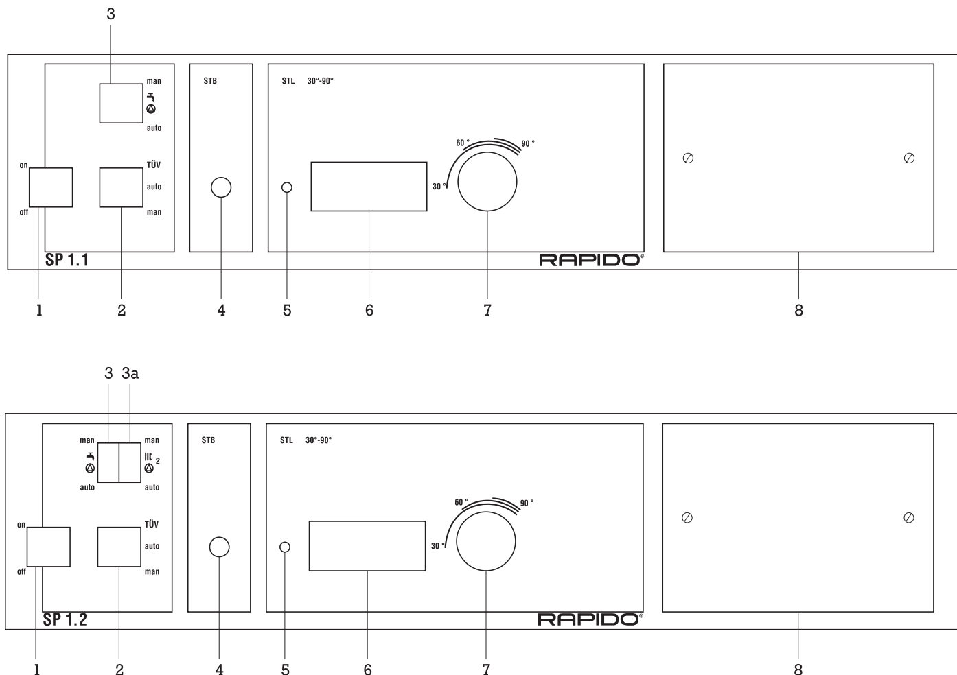
Рис. 8 Вид спереди панели управления SP 1.1 и SP 1.2
