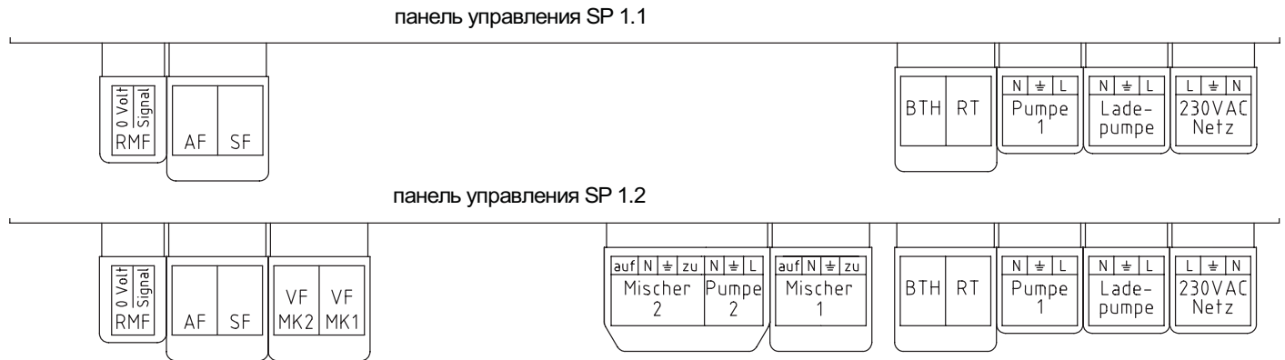
Рис. 6.1 Контакты электрических соединений
