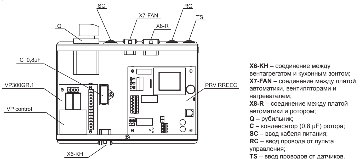
Рис. 4 Клеммная коробка вентагрегата.
