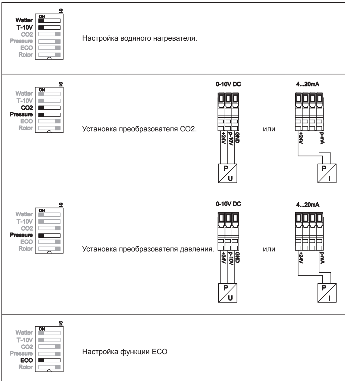
Рис. 3 Значение микропереключателей S1.
