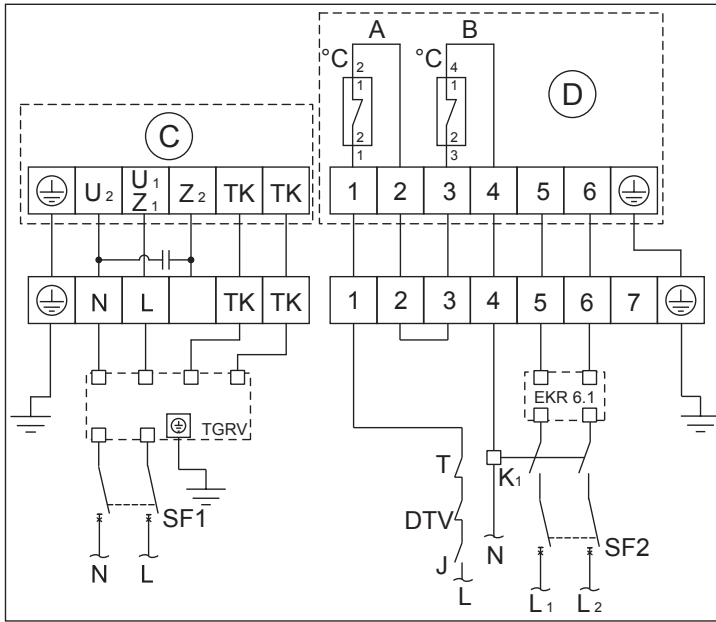
Схема подключения № 10
