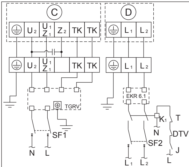
Схема подключения № 6
