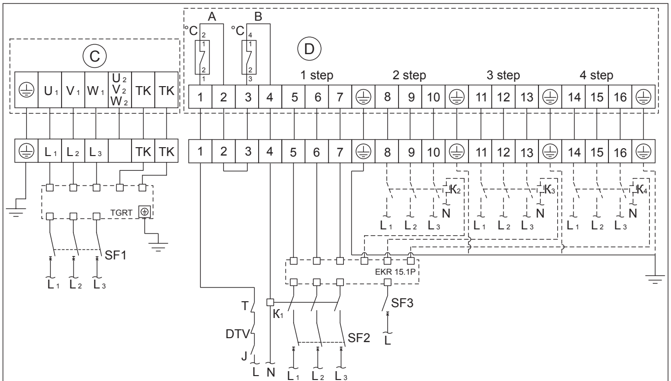
Схема подключения № 13
