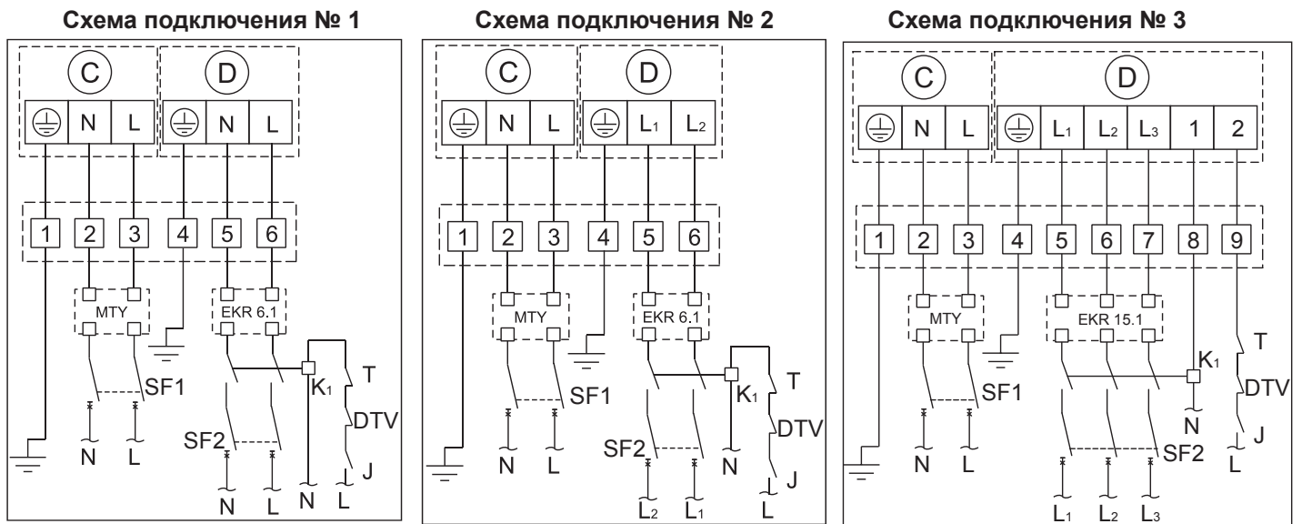
Рис. 1 Электрические схемы № 1-3.
