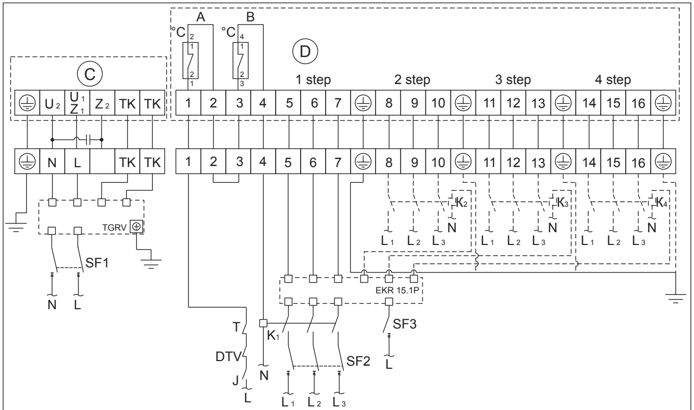
Схема подключения № 13
