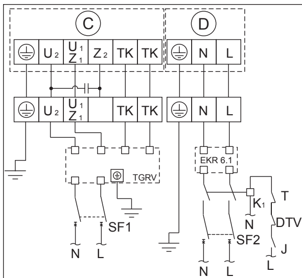
Рис. 2.1 Электрические схемы № 4-9.
