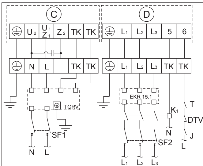
Схема подключения № 8
