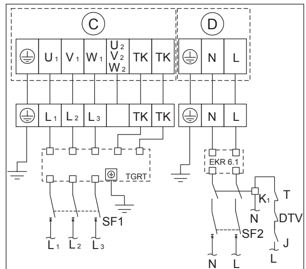
Рис. 2.1 Электрические схемы № 4-9.
