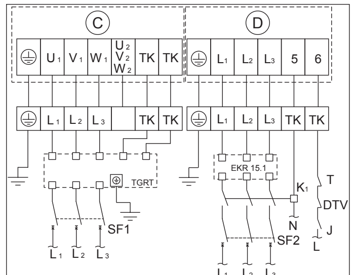
Схема подключения № 9
