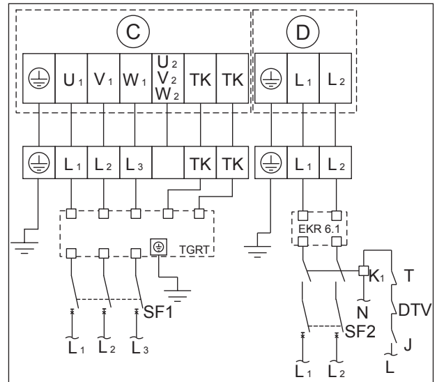
Схема подключения № 7
