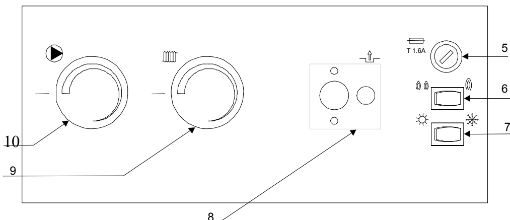
Рис.36 Панель вертикальная
