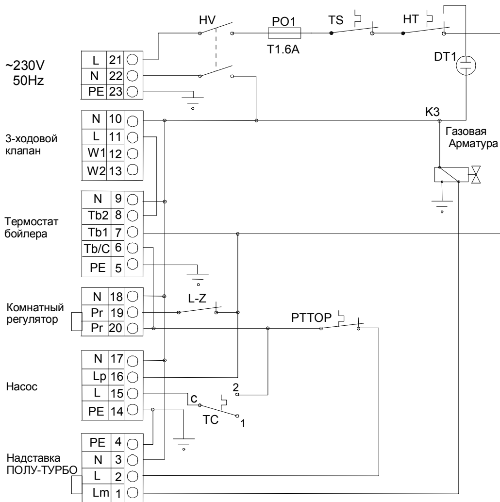
Рис. 56 – Схема электрического подключения котла 60 PLO
