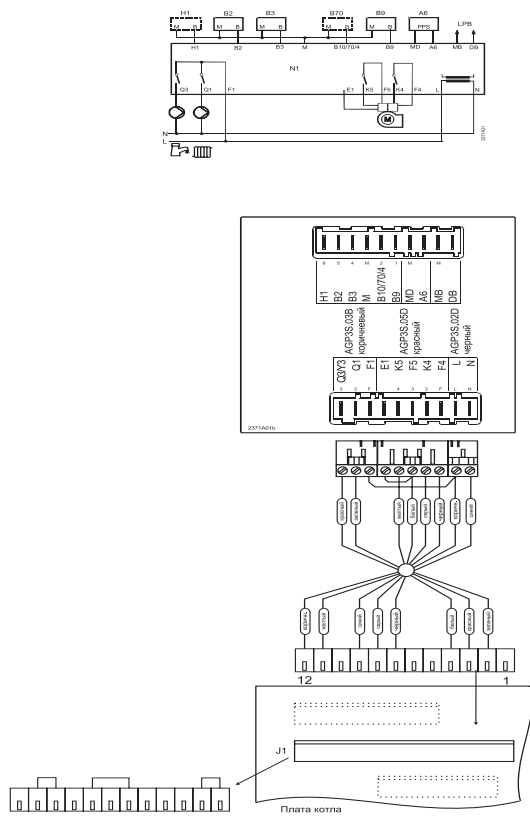
Схема подключения присоединительного комплекта для котла КЛО и регулятор RVA 43-222
