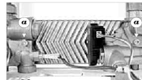
Рис. 24 - Теплообменник
