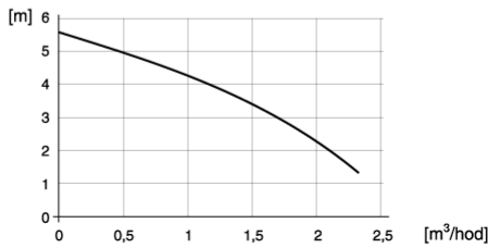
Рис. 5 – Характеристика насоса
