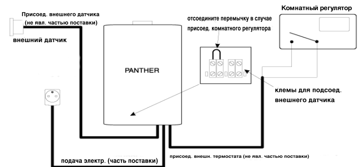
Рис. 15 – Эл.подсоединение термостата и внешнего датчика
