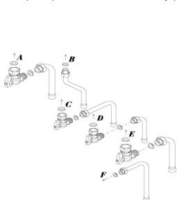
Рис. 8 – Присоединительный комплект медных трубок
