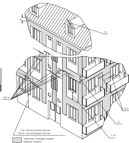
рис.21 Размещение на фасад
