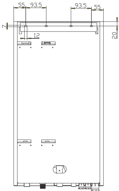
Вид сзади
