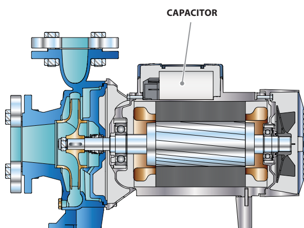
Однофазная версия
