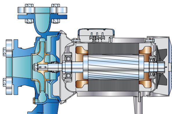
Трехфазная версия
